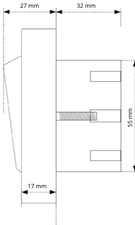
zijaanzicht
